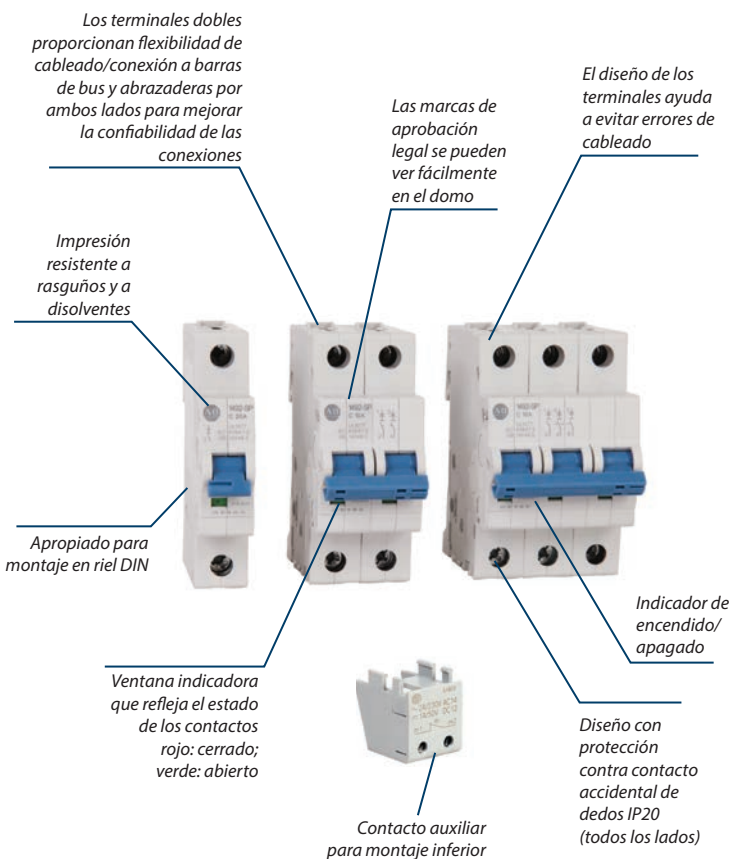
Protección de circuitos de control y de carga
