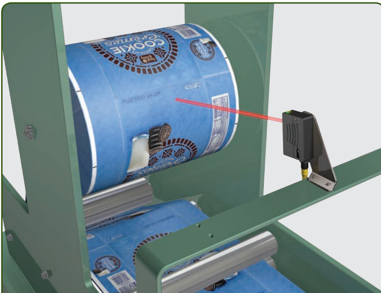
Diámetro de rollo – Un sensor 45LMS mide el diámetro de un rollo para controlar su velocidad y prevenir su desvío.
