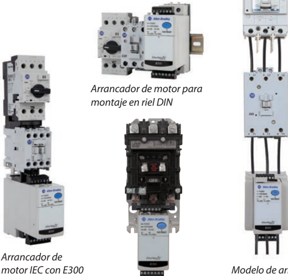
Arrancador de motor NEMA con E300
