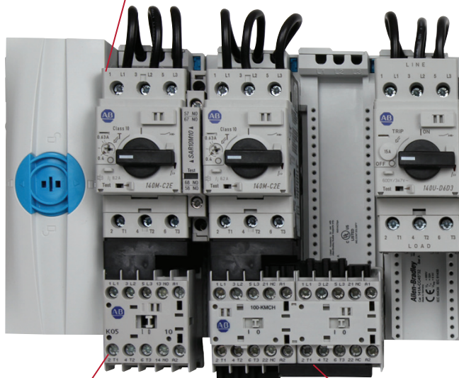
Disyuntor de protección de motor 140M
