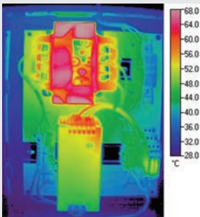
A-B 1606-XLS – 10 A, 24 VCC – Eficiencia de 93%
