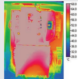
Competencia B – 10 A, 24 VCC – Eficiencia de 84%
