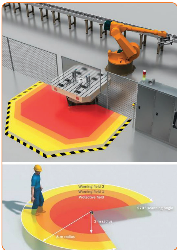
Dispositivos de detección de presencia
