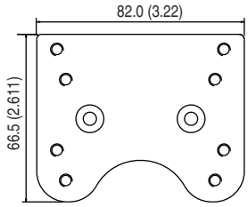
440J-A03N Double Actuator Plate
