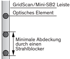
Abb 9: Torausblendung durch Torunterkante
