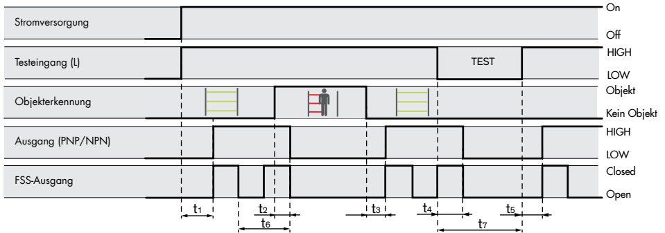
Abb 14: Zeitdiagramm
