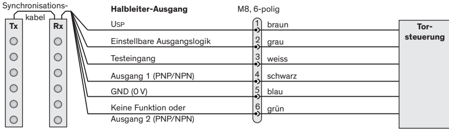
Abb 11: Anschlussdiagramm Halbleiter-Ausgang
