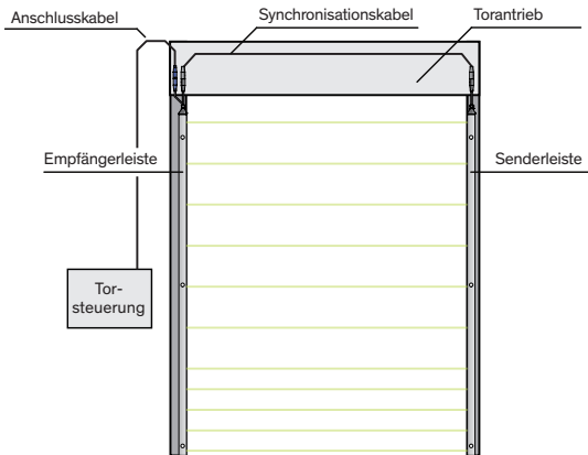
Abb 6: GridScan/Mini-SB2/-ST2 Anwendungsübersicht
