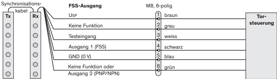
Abb 12: Anschlussdiagramm FSS-Ausgang
